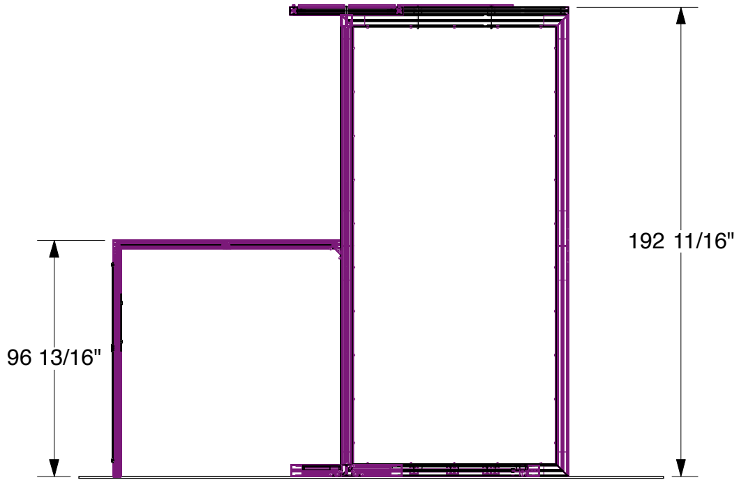
ELEVATION
